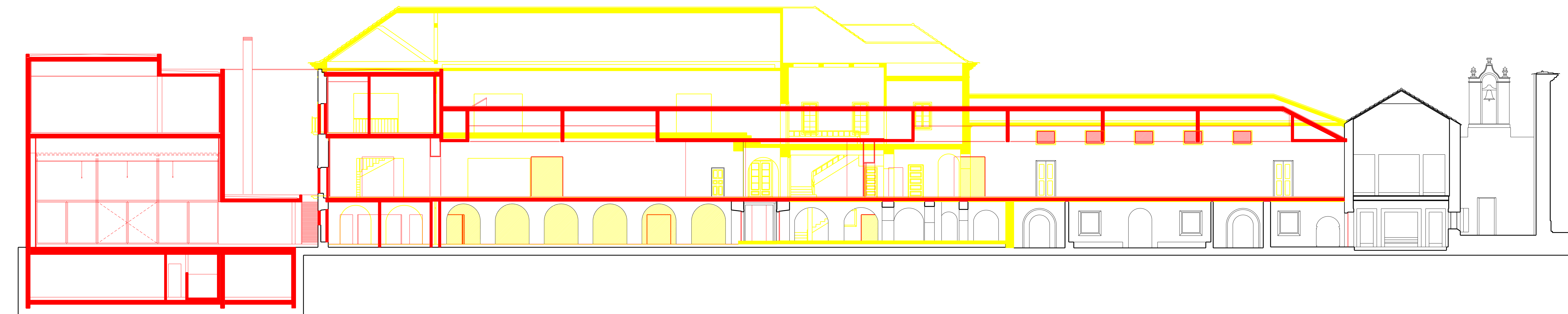
CORTE 3
