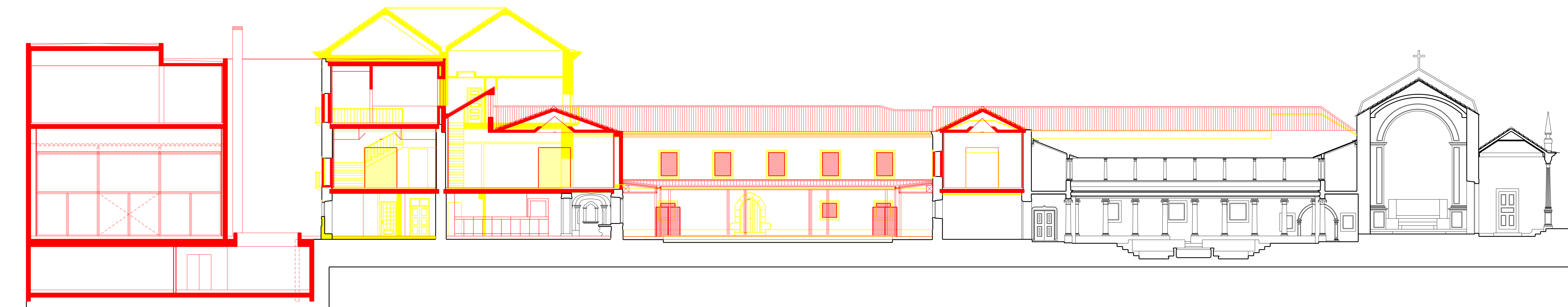
CORTE 4
