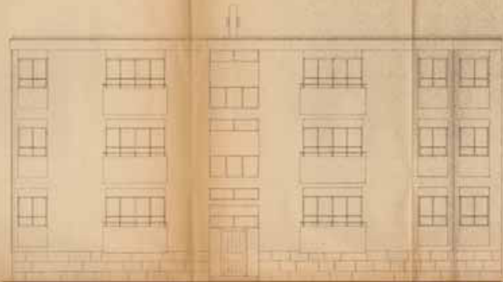
ALÇADO PRINCIPAL
