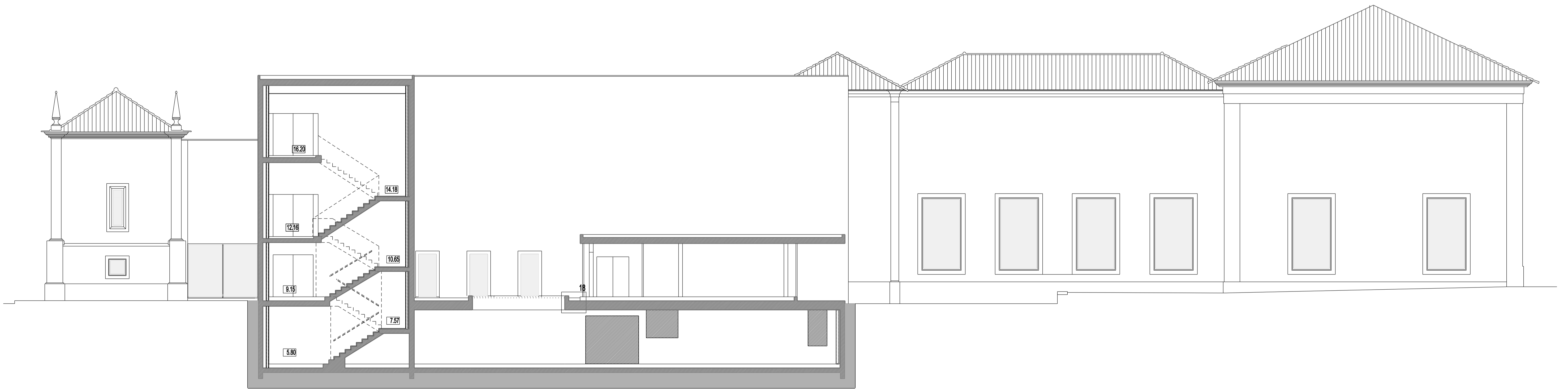
CORTE 10
