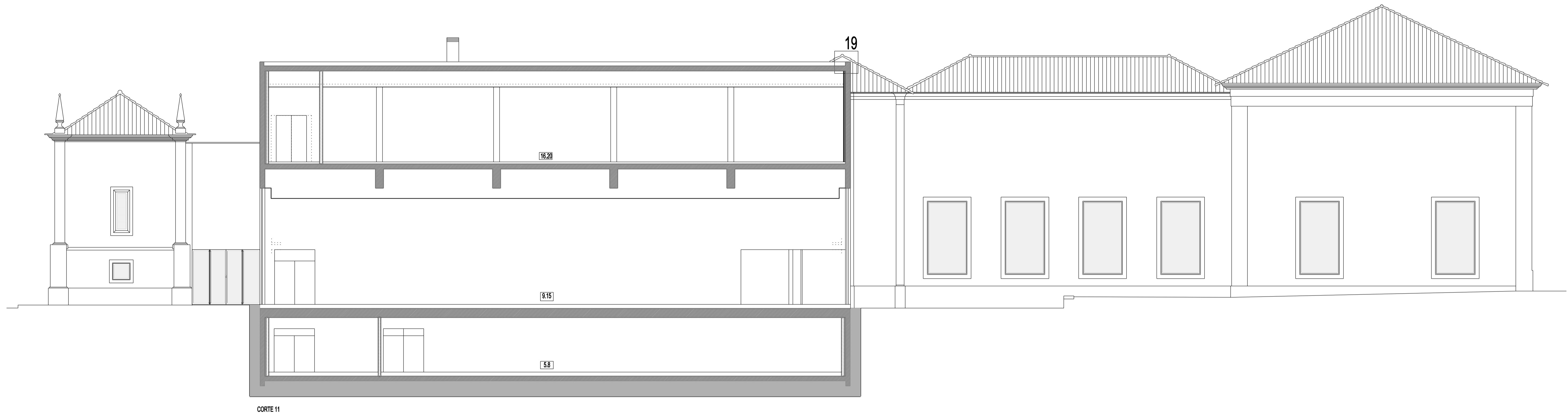
CORTE 11
