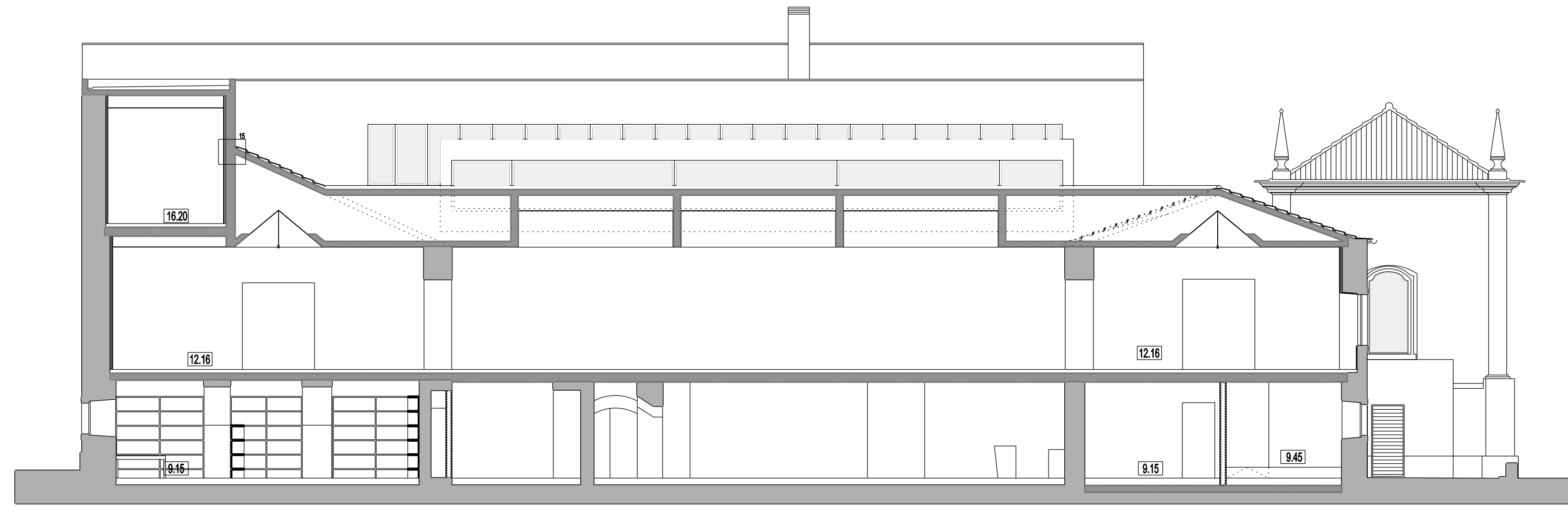
CORTE 5
