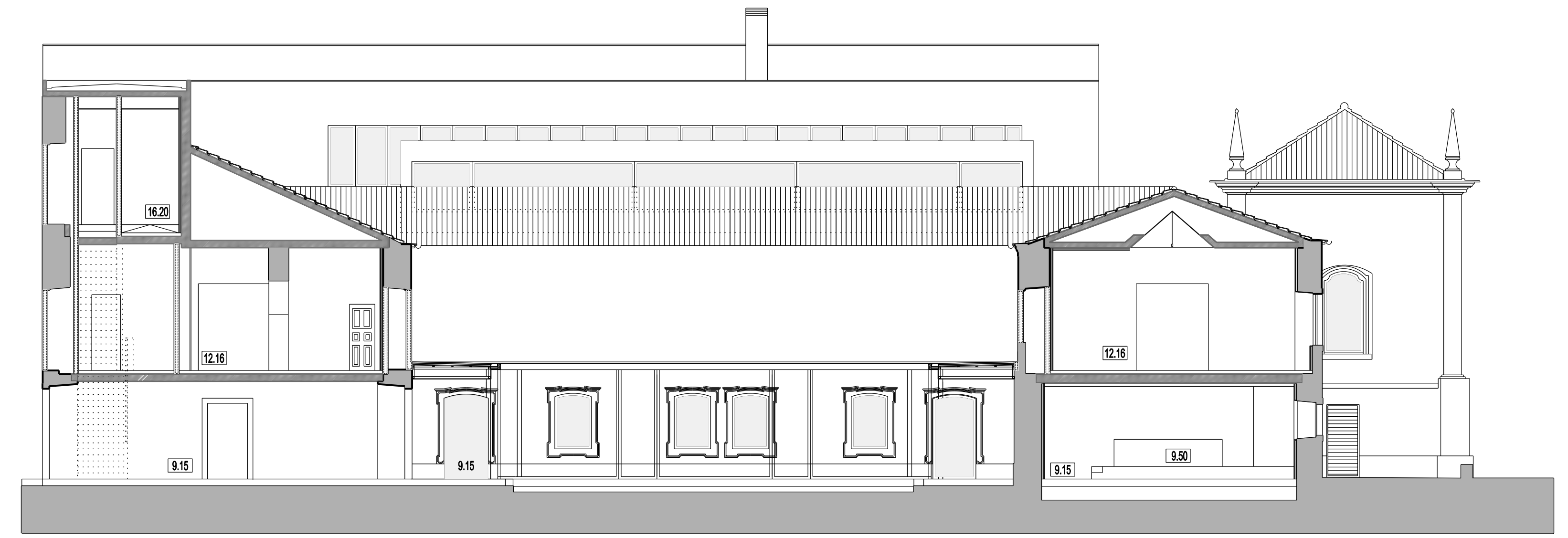
CORTE 6
