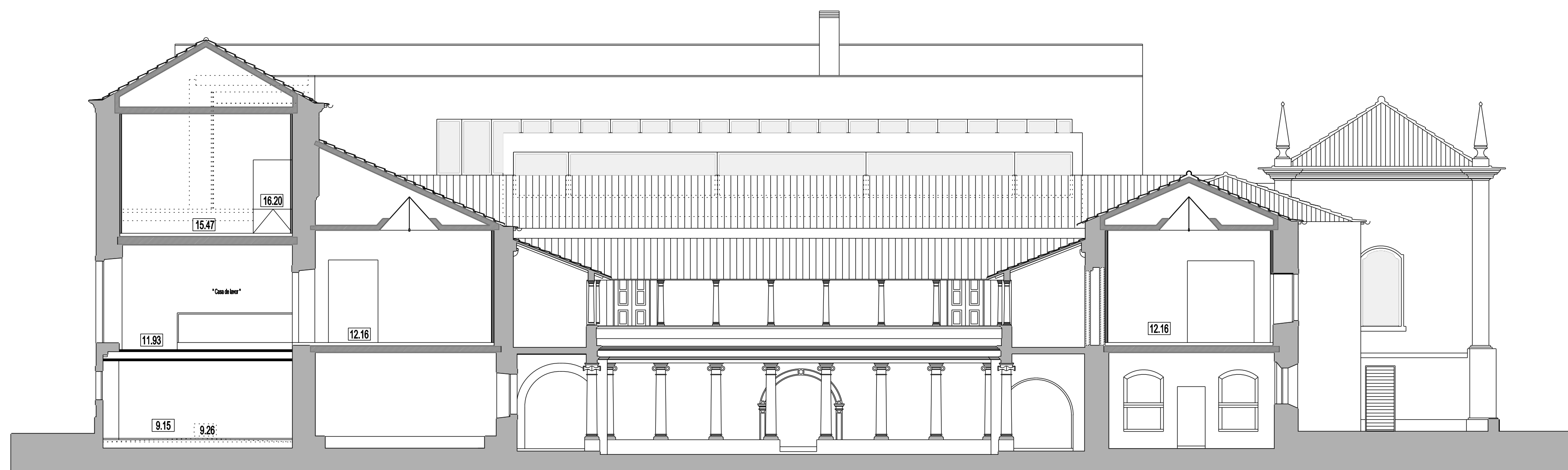
CORTE 7
