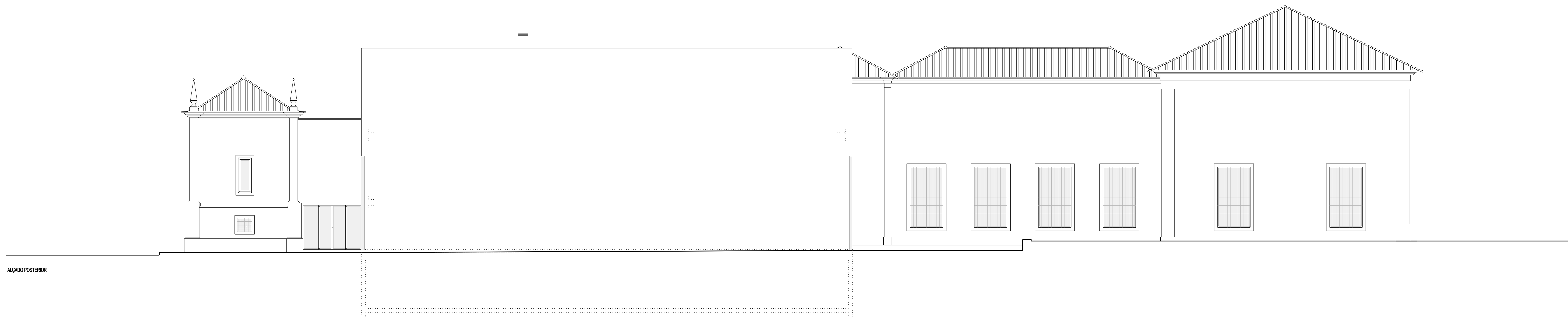
ALÇADO LATERAL ESQUERDO
